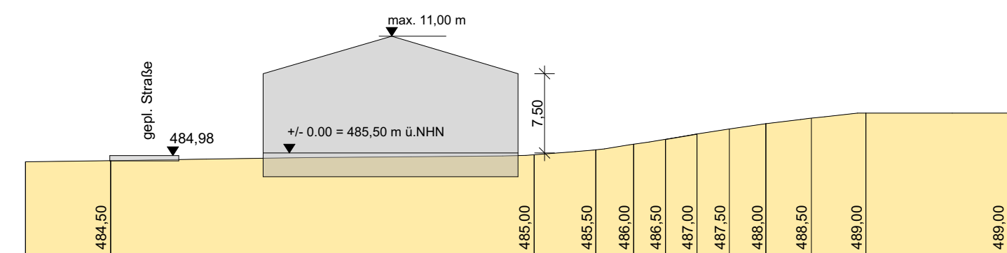
Schnitt 5-5 Parz. 6
