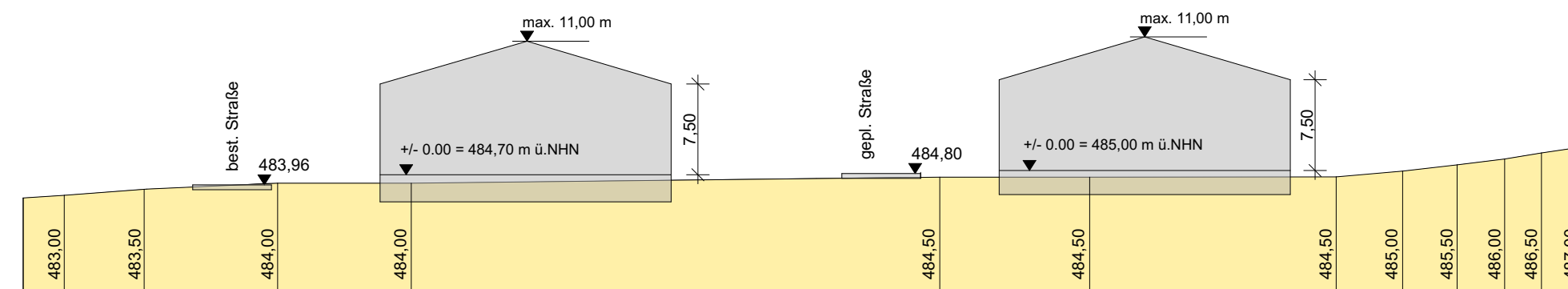
Schnitt 4-4 Parz. 10 Parz. 5
