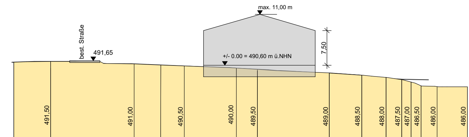
Schnitt 11-11 Parz. 16 b
