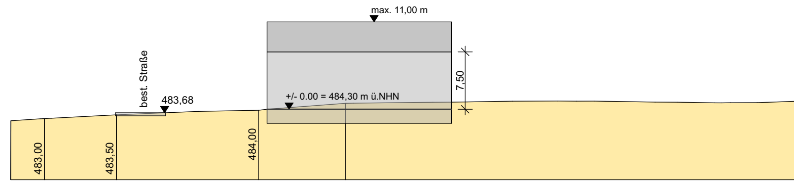
Schnitt 1-1 Parz. 1
