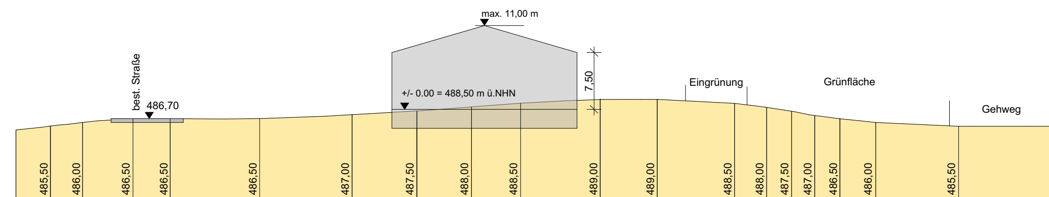
Schnitt 9-9 Parz. 15
