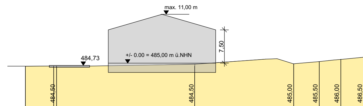
Schnitt 3-3 Parz. 4
